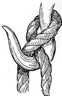
FIG. 45.—Blackwall hitch.
